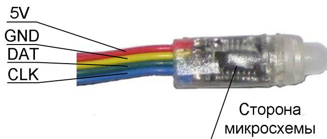
Маркировка проводов
